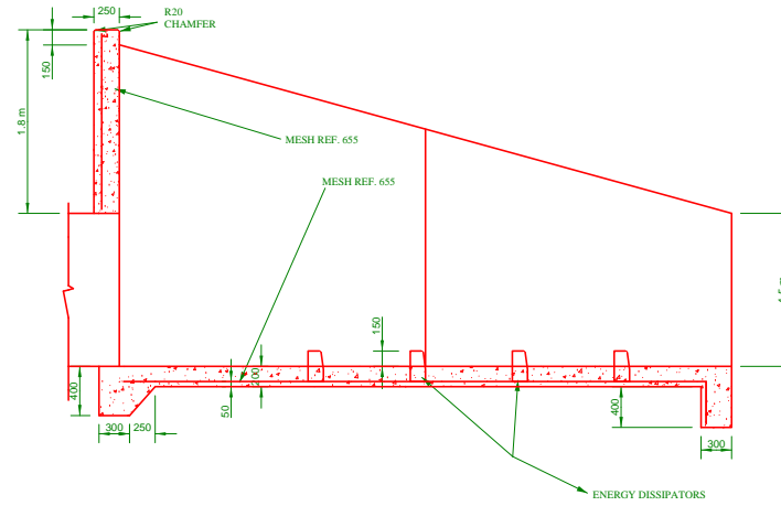
SECTION A-A Scale 1:35
